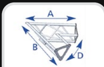
ASX42 A : 710B : 500 C : 500D : 90°
