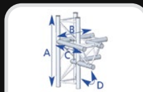
ASX45 A : 742B : 500 C : 500D : 90°
