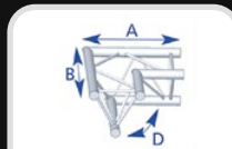
ASX22 A : 500B : 500 C : /D : 90°
