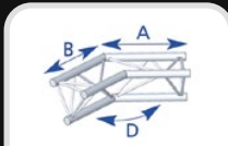
ASX25 A : 500B : 500 C : /D : 135°
