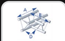
ASX33 A : 710B : 500 C : /D : 90°
