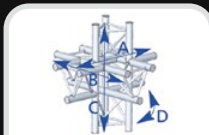
ASX61 A : 710B : 710 C : 742D : 90°
